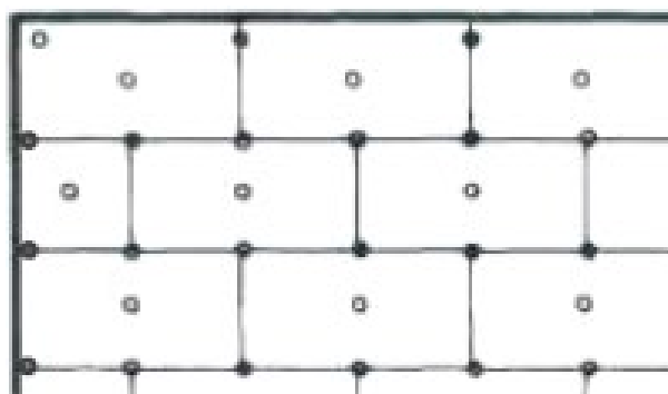
Montageschema 1: Befestigung in der Plattenmitte und an den T-Stößen
