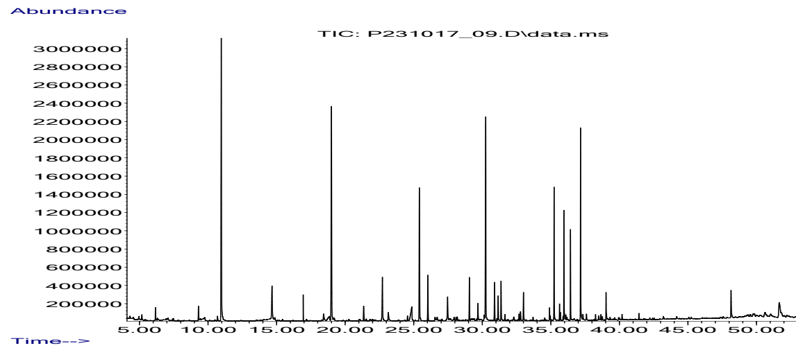
Chromatogramm Tag 3
